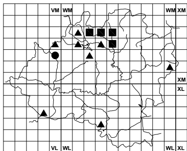
Arabis glabra
