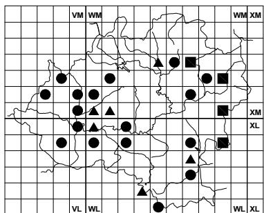
Alyssum serpyllifolium
