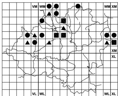
Arabis alpina
