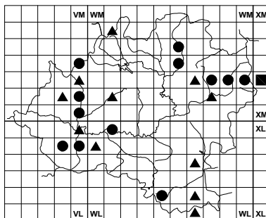
Alyssum montanum
