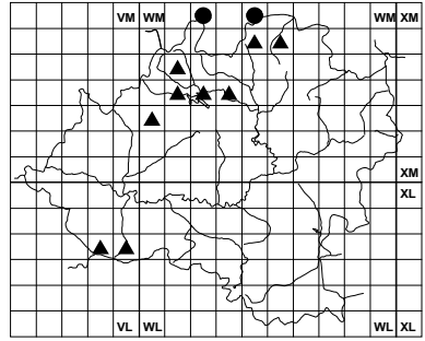
Hieracium sabaudum
