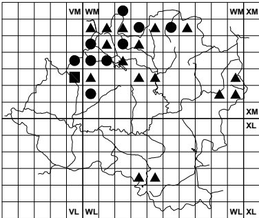
Hieracium schmidtii
