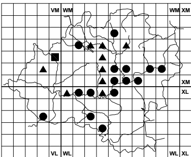
Hypochaeris glabra
