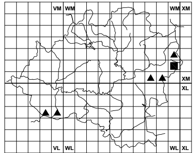
Hieracium segurae
