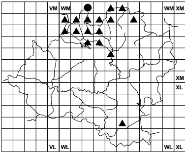
Hieracium maculatum
