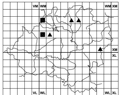
Hypochaeris maculata
