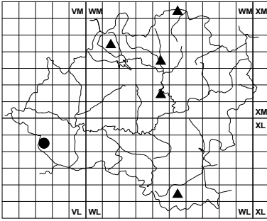
Hieracium pulmonaroides
