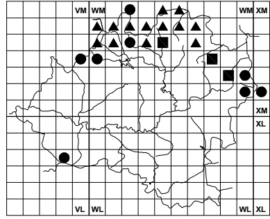
Hieracium murorum
